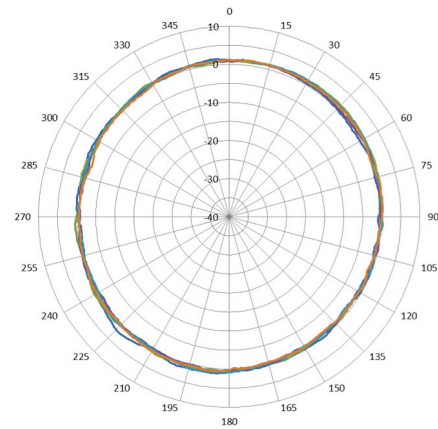
H-plane – 5 GHz
