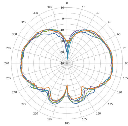
E-plane – 5 GHz
